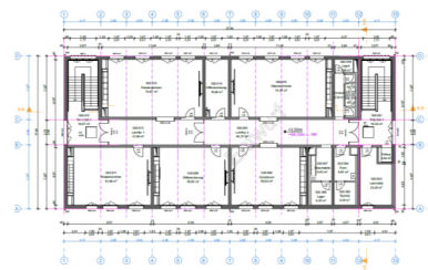
Grundriss OG
