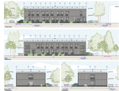
Ansichten
