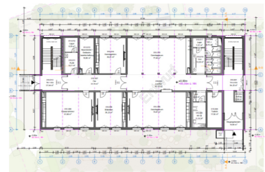
Grundriss EG
