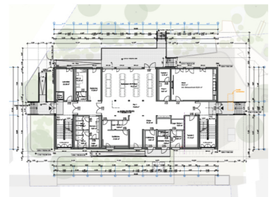
Grundriss EG
