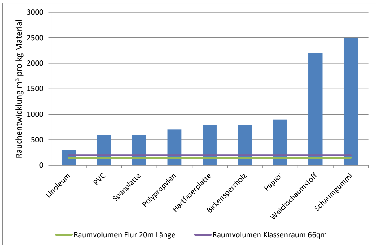
Abbildung 1 - Rauchentwicklung (Rauchvolumen pro Kg brennbarem Material)
