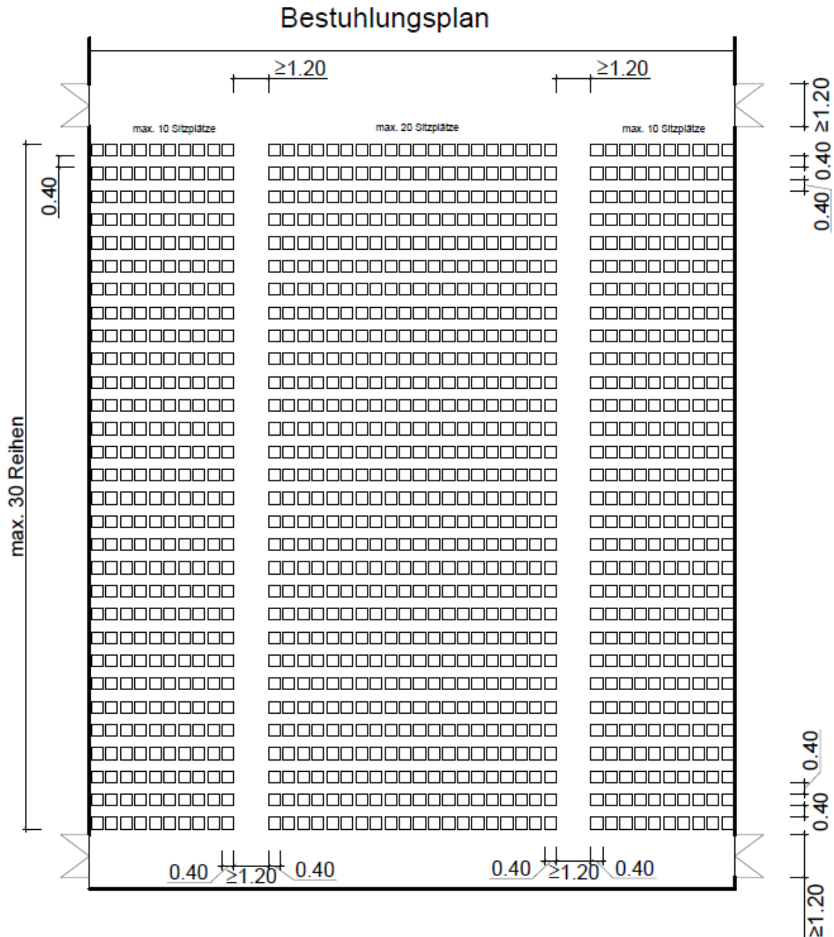
Abbildung 15 - Beispiel Bestuhlungsplan mit maximaler Blockgröße und Minstdurchgangsbreite
