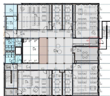
Ausschnitt Grundriss Lerncluster
