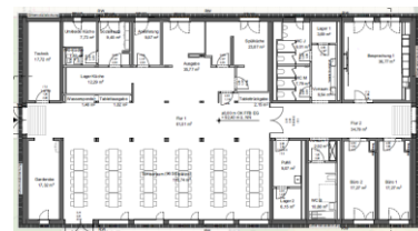
Grundriss EG
